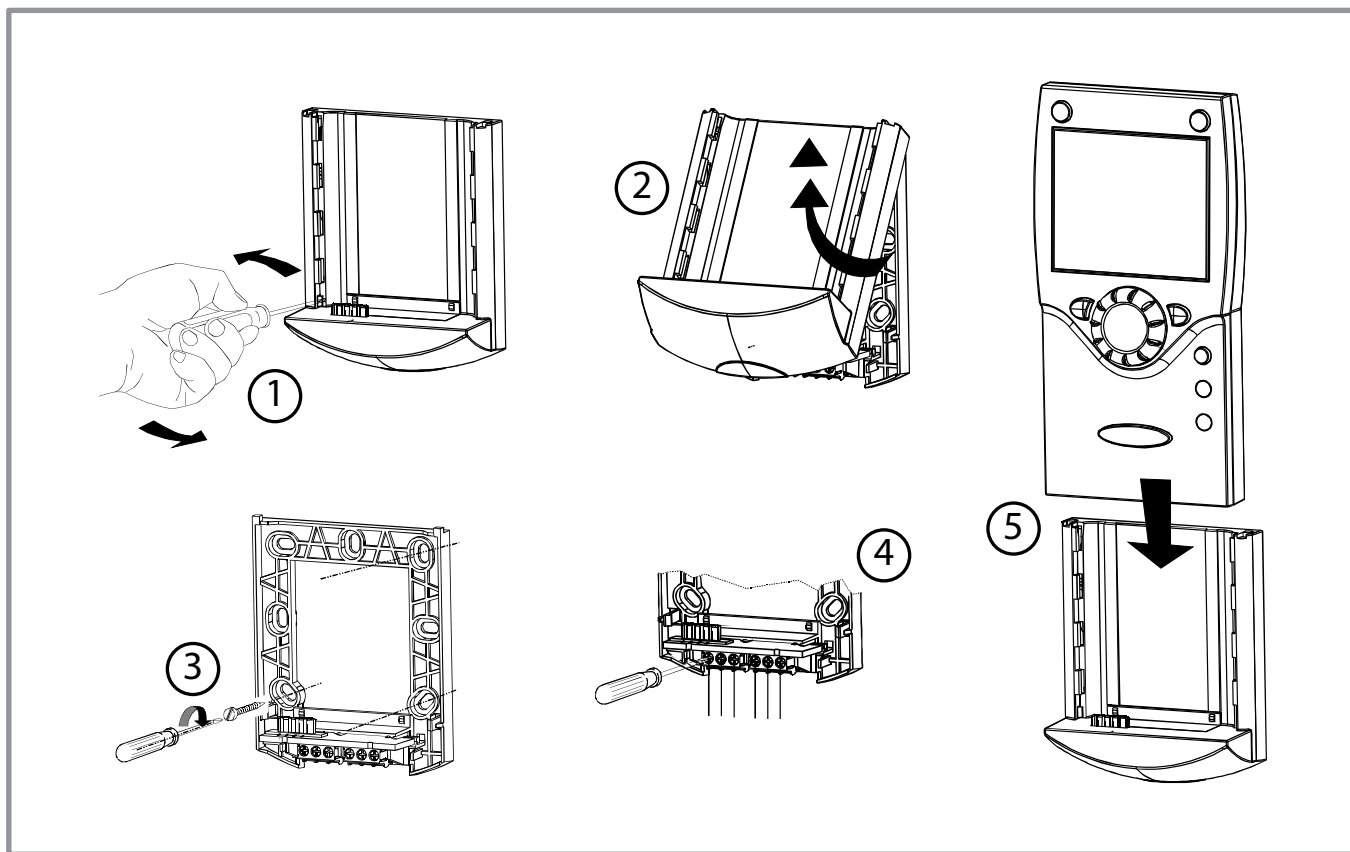
figure 5 - Montage avec socle
