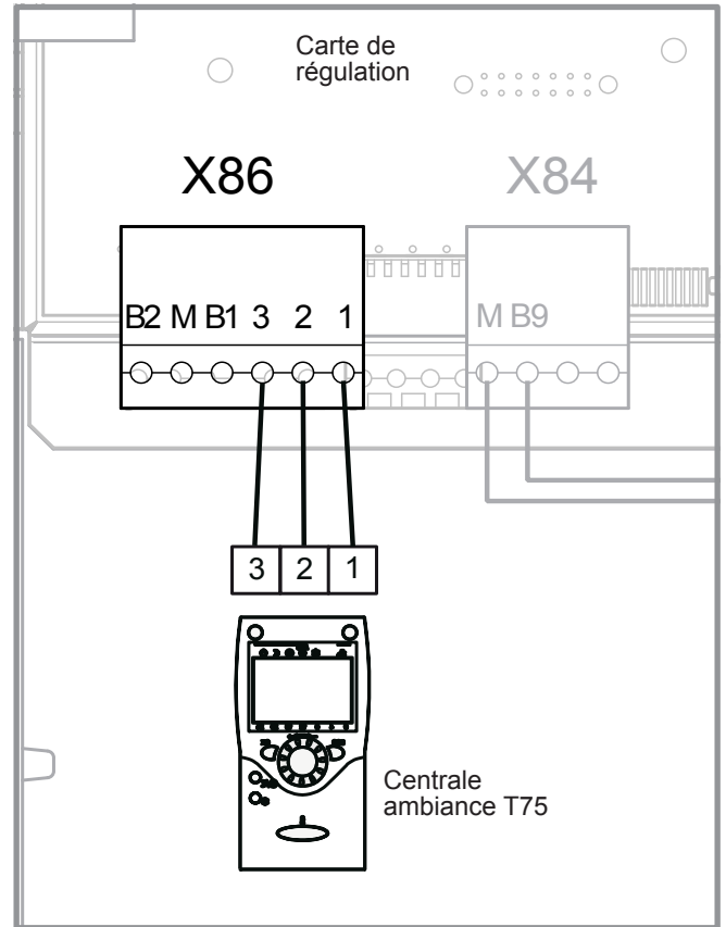
figure 6 - Raccordement sur la carte de régulation
