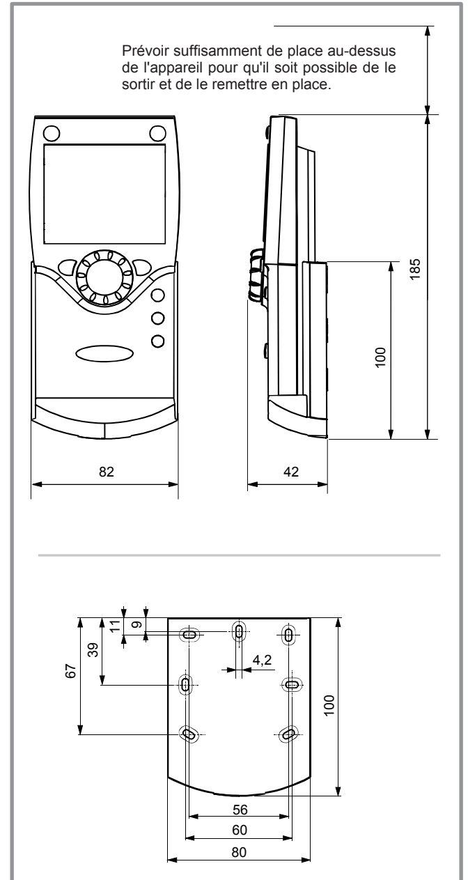
figure 3 - Dimensions en mm
