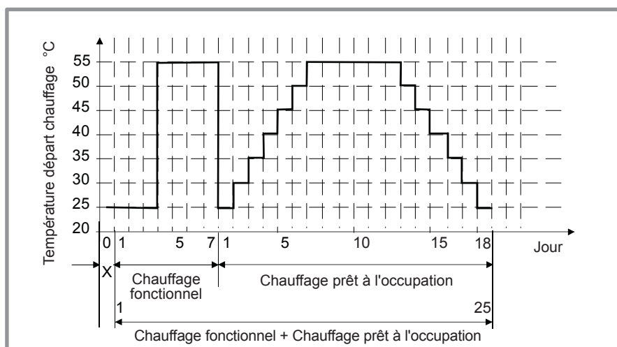
figure 9 - Diagramme des programmes de séchage de dalle
