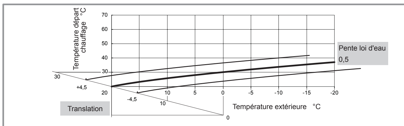
figure 8 - Translation de la courbe de chauffe (ligne 721)
