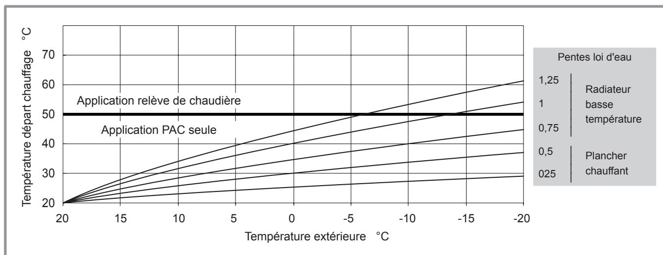
figure 7 - Pente de la courbe de chauffe (ligne 720)
