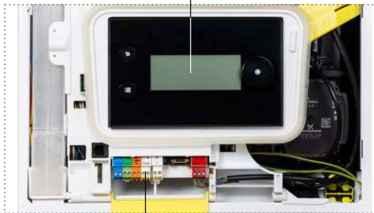
Bornier à vis de raccords électriques Emplacement pour carte électronique d'extension SCB 17
