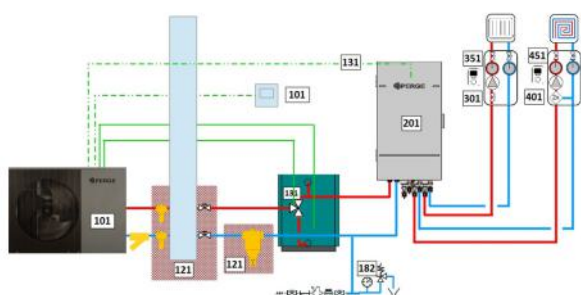
OptiPac MR290 couplée à une chaudière fioul existante
